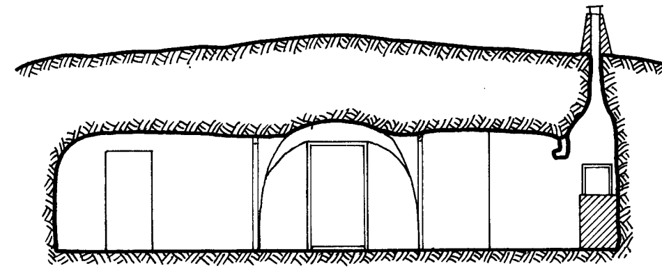
SECCIÓN B-B
